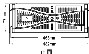
正面
