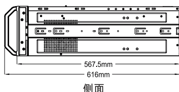
侧面
